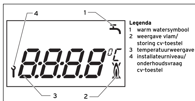
Afb. 1.2 Overzicht display
