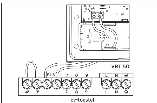
Afb. 9.1b Elektrische aansluiting NL
